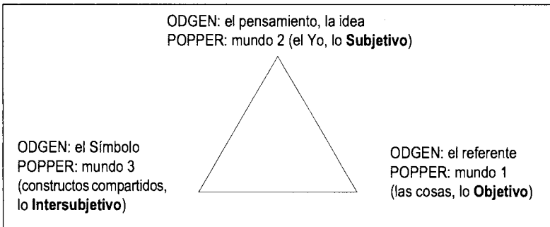
Gráfico 1: Triángulo de Odgen y los 3 mundos de Popper
