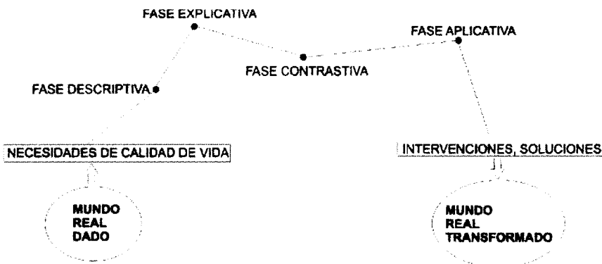
Gráfico 2: Estructura Diacrónica de los Procesos de Investigación
